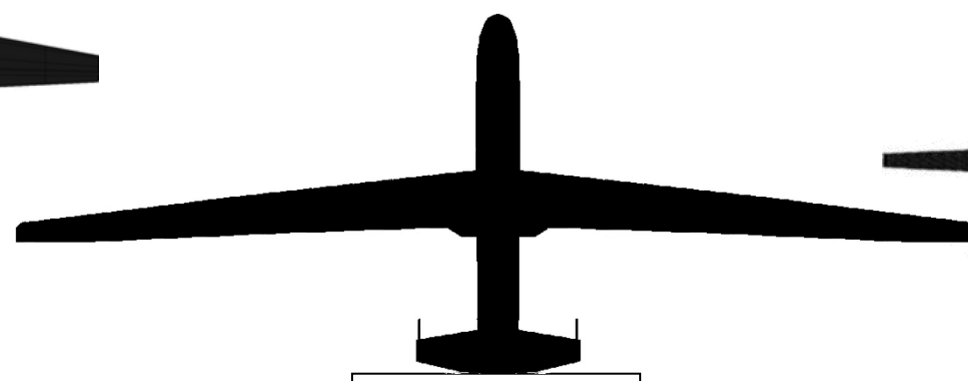
RQ-4 Global Hawk W: 39.8m L: 14.5m
